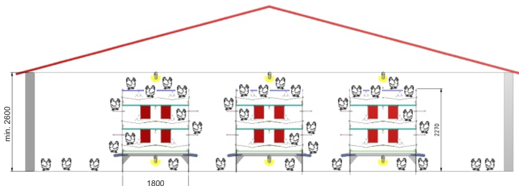
Příklad umístění voliérového systému
