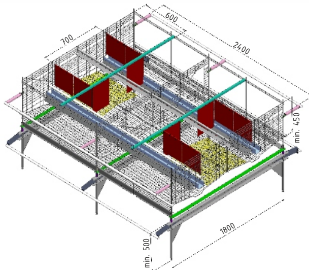
Rozměry alternativního modulu
